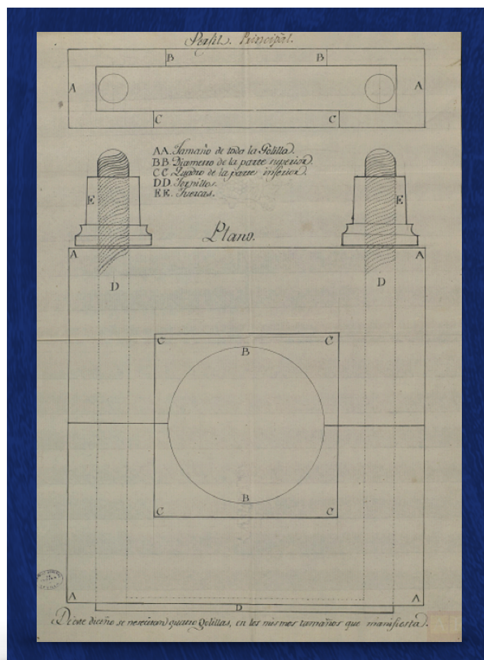
Plano y perfil de la golilla para volante de máquina de cortar moneda que se debe enviar a la Casa de Moneda de Santa Fe, 19/09/1796, Archivo General de Indias, MP-Ingenios, 287BIS
