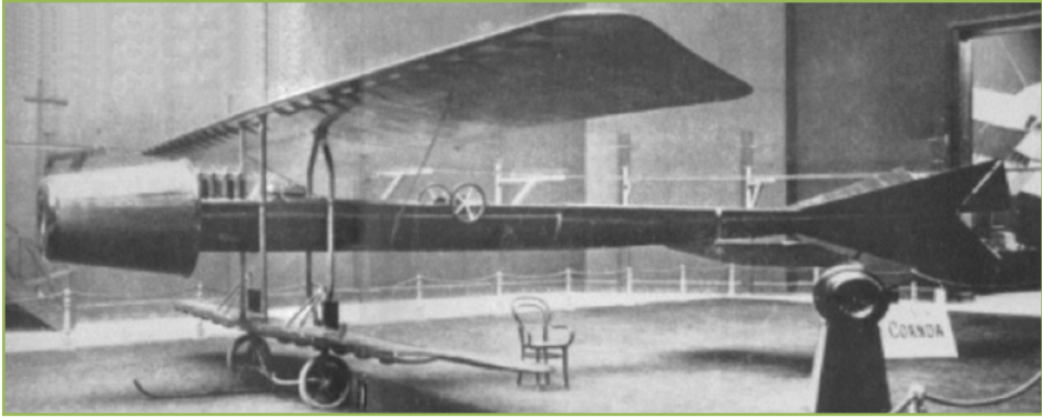
El Coandă-1910, el primer avión construido con un motor de reacción
