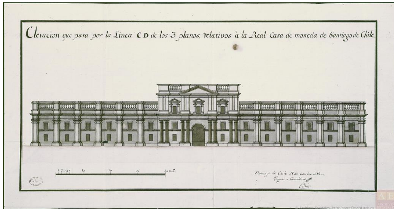
Elevación que pasa por la línea CD de los Tres planos relativos a la Real Casa de Moneda... de Santiago de Chile. Archivo General de Indias, MP-PERU CHILE, 242
