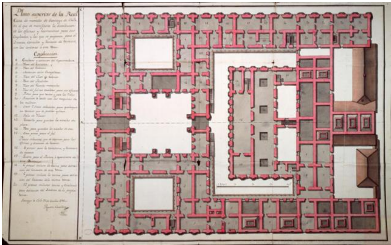
Plano superior de la Real Casa de Moneda de Santiago de Chile... Archivo General de Indias, MP-PERU CHILE, 239
