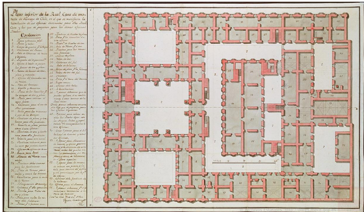
Plano inferior de la Real Casa de Moneda... de Santiago de Chile Archivo General de Indias, MP-PERU CHILE, 240
